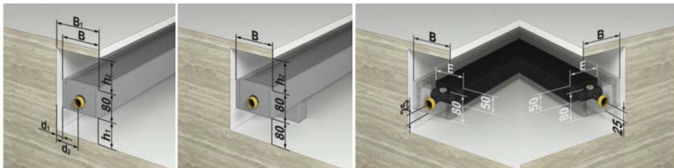
Настенный монтаж
