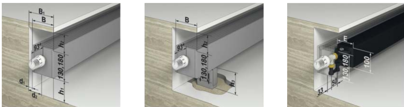
Настенный монтаж
