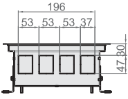
Вид с торца Ntherm 250.110
