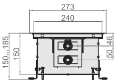
Разрез Ntherm 250.150
