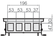
Вид с торца Ntherm 250.90
