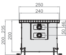
Разрез Ntherm 250.200
