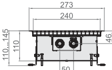
Разрез Ntherm 250.110
