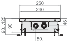
Разрез Ntherm 250.90
