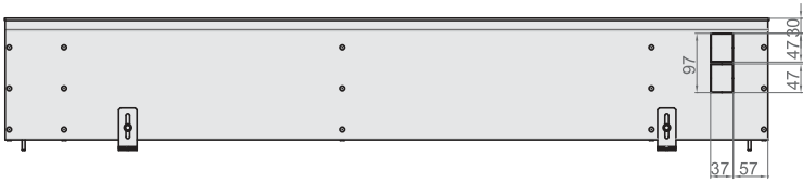
Вид сбоку конвектора Ntherm 250.200 с U-образным бортом.
