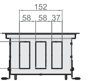
Вид с торца Ntherm 250.150
