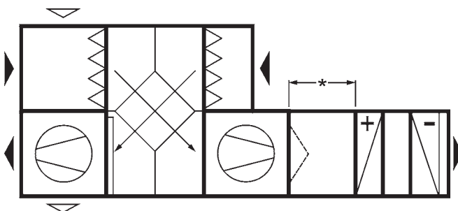
горизонтально, один на другом, с перекрестноточным рекуператором
