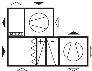
горизонтально, один на другом, с перекрестноточным рекуператором
