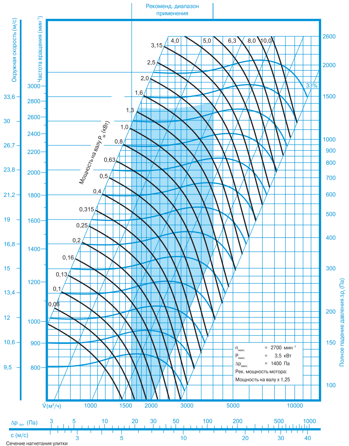
Диаграмма вентилятора
