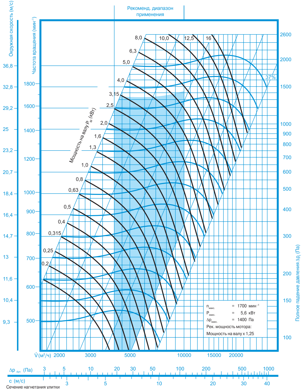
Диаграмма вентилятора
