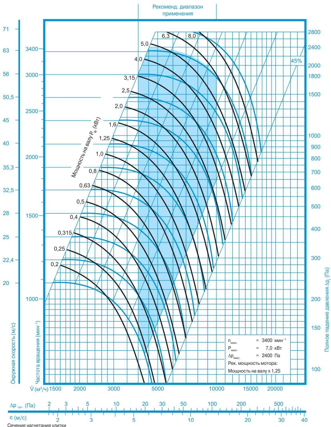
Диаграмма вентилятора
